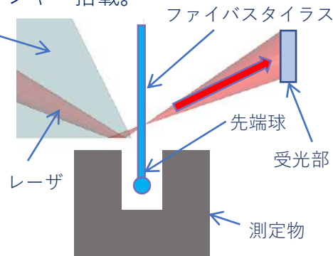
スタイラス先端拡大図
