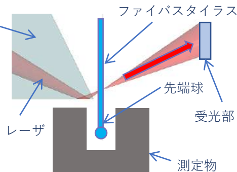
スタイラス先端大図
