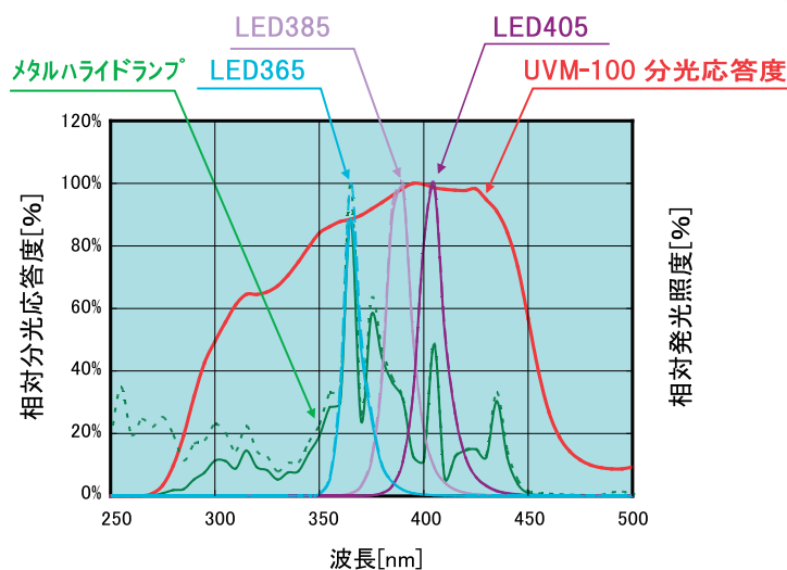
センサ部の相対分光応答度特性（代表値）
