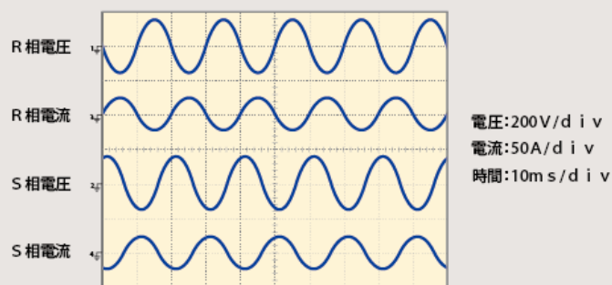
動作電源の入力電圧・電流波形
