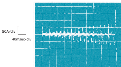
防止回路がついている電源
