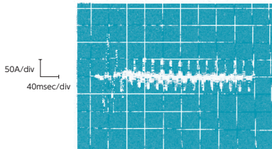
防止回路のない電源
