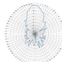
28GHzビームパターン
