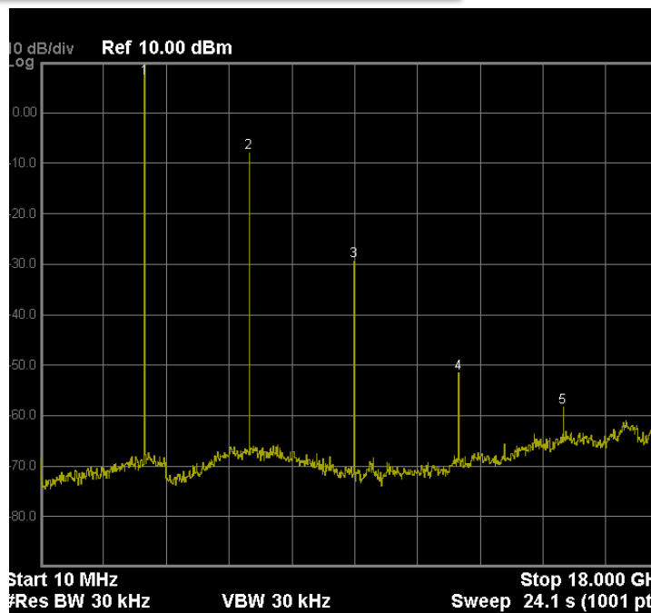
▲高調波画像 (周波数 3.0GHz時)
