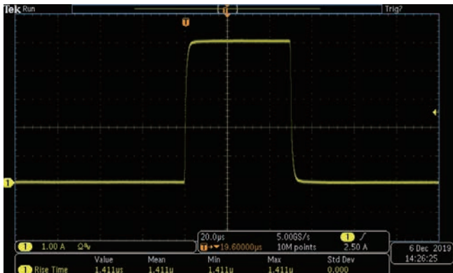
2601B-PULSE型による出力。オーバーシュートはなく、立上り時間は 1.4\mu\text{s} 。
