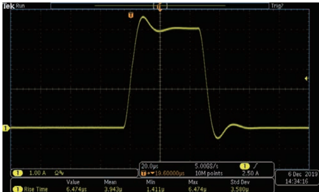
他社製品のソースメータによる一般的なパルス出力。オーバーシュートが発生し、立上り時間は 6.47\mu\text{s} となっている。
