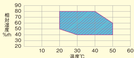
温湿度制御マトリクス
